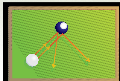
Figura 2. Fixando uma segunda bola à mesa, obtemos o chamado bilhar de Sinai. A segunda bola desfocaliza as trajetórias da primeira, gerando um movimento irregular ou caótico.
