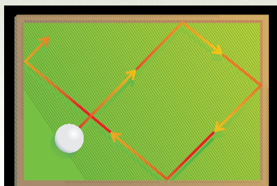
Figura 1. Um bilhar formado por uma só bola e mesa retangular sem caçapas não é caótico. Depois de quatro colisões com a borda, a trajetória da bola volta a ter a mesma direção.
