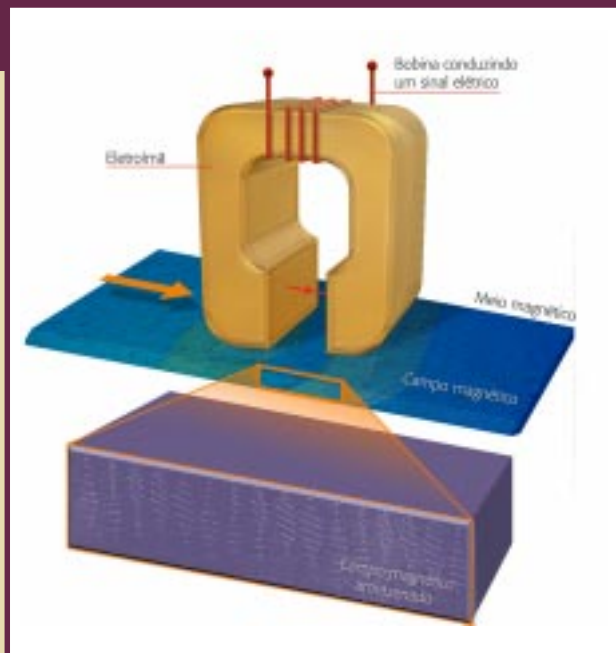
Figura 1. Esquema mostra como ocorre a gravação em meio magnético. O sinal elétrico que chega à bobina induz no eletroímã um campo magnético que, por sua vez, é responsável por armazenar (gravar) no meio magnético a informação transportada pelo sinal.
