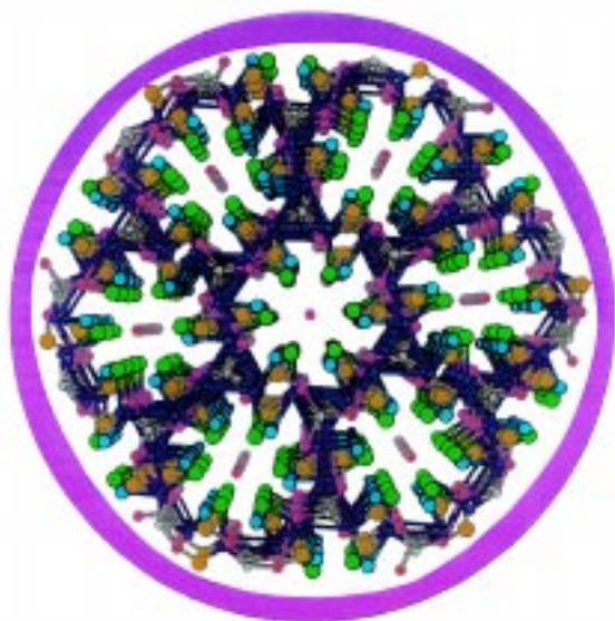
Figura 4. Visão superior de um conjunto de 1.800 átomos da hidroxiapatita, principal componente mineral dos ossos e esmalte dentário. As esferas verdes e cinzas são átomos de cálcio. As esferas laranjas são os átomos de fósforo. Todas as outras esferas representam os átomos de oxigênio e hidrogênio.
