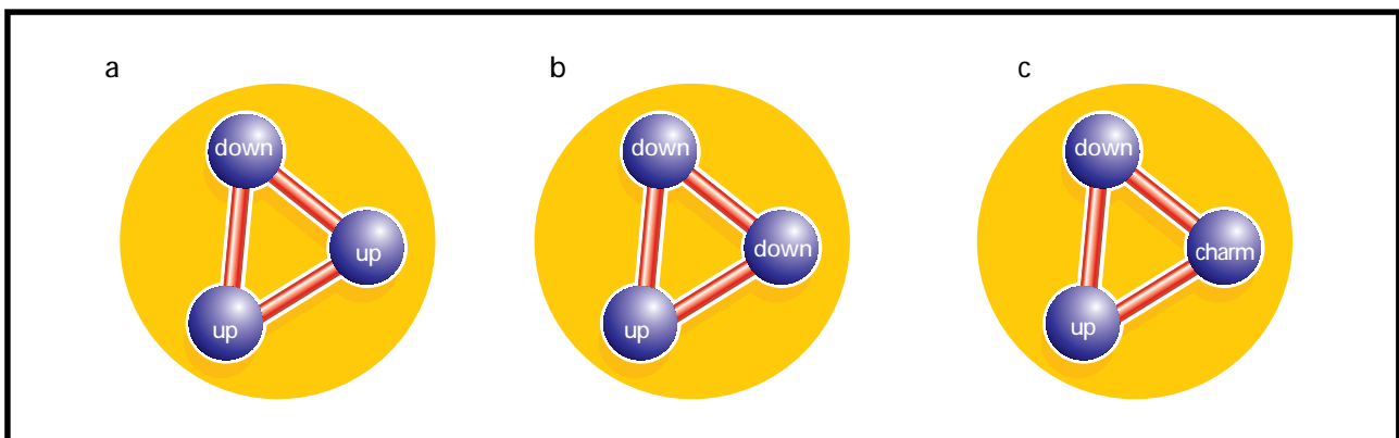
Figura 1. Exemplos de bárions, partículas formadas por três quarks. Em a, representação de um próton (componente do núcleo atômico), que tem carga elétrica +1 e é formado por dois quarks up (carga elétrica +2/3) e um quark down (-1/3). Em b, um nêutron, outro componente nuclear, que tem carga elétrica nula, sendo formado por dois quarks down (-1/3) e um up (+2/3). A combinação dos seis quarks existentes pode formar várias outras partículas, como o lambda (item c), constituído por um up , um down e um quark charm , este com carga elétrica +2/3. Partículas formadas por um dupla de quarks são denominadas mésons. Um exemplo são os glúons (aqui representados pelas linhas que unem os quarks), que podem momentaneamente formar um par quark e antiquark.
